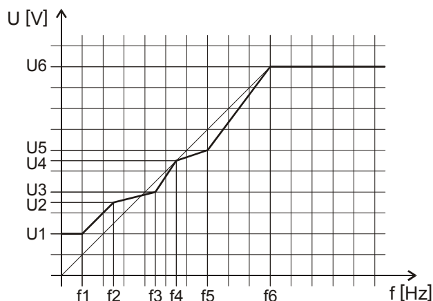
Tetszőleges U/f felhasználói-karakterisztika
