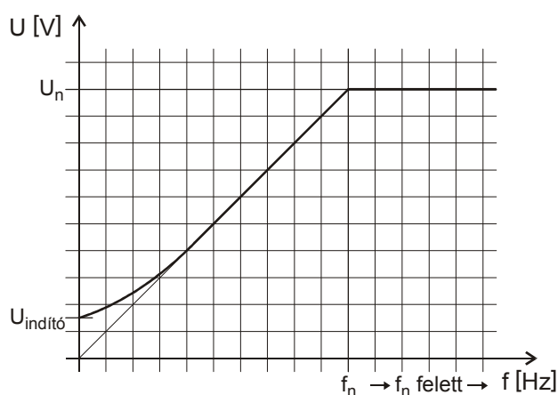
Lineáris U/f felhasználói-karakterisztika
