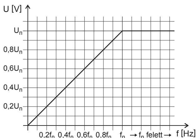
Lineáris U/f alap-karakterisztika
